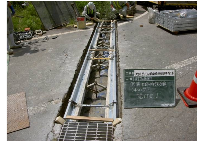
7. 側溝上部補強金具据付完了
